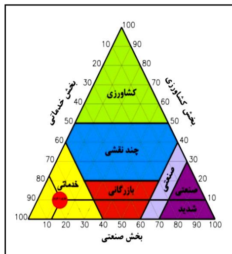
شکل ۲. مثلث بوژوگارنیه
