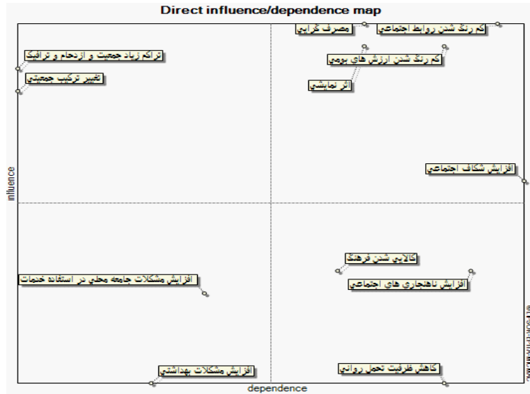
شکل ۱۱. نمودار تأثیرگذاری و تأثیرپذیری مستقیم اثرات منفی اجتماعی- فرهنگی
