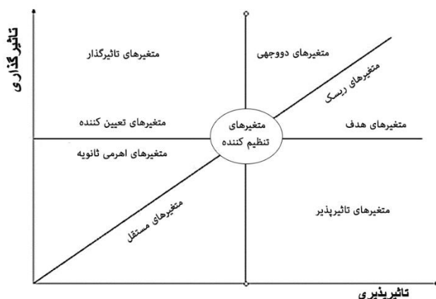
شکل ۳. نمودار پراکندگی متغیرها از نظر تأثیر پذیری و تأثیر گذاری. منبع: بهشتی و زالی (۱۳۹۰: ۴۷)
