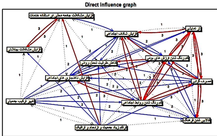
شکل ۱۲. گراف تأثیرگذاری مستقیم اثرات منفی اجتماعی- فرهنگی
