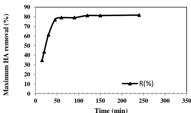
شکل ۳. اثر زمان تماس بر جذب اسید هیومیک (غلظت آلاینده ۵۰ میلی گرم در لیتر، دوز جاذب ۰/۱ گرم در لیتر و pH=7 ).
