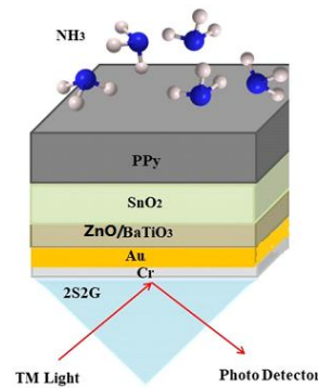
شکل ۱- ساختار حسگر SPR پیشنهادی برای تشخیص NH_3 بر اساس لایه‌های PPy و SnO_2 ، BaTiO_3 ، ZnO
