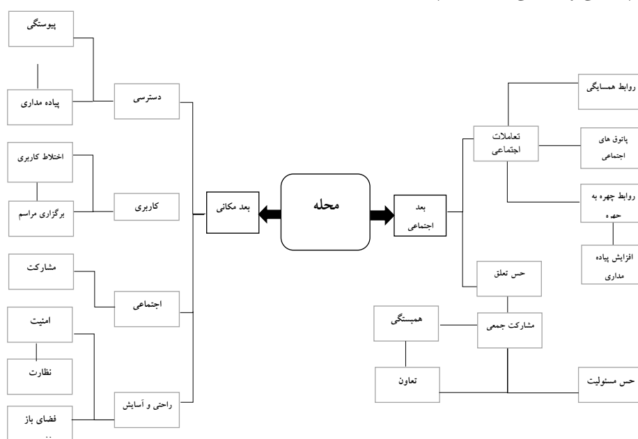
شکل ۱- دیاگرام ابعاد تأثیرگذار بر روابط اجتماعی در محله، (منبع: نگارندگان)
