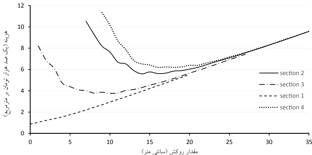
شکل ۳. نمودار هزینه کلی نسبت به ضخامت روکش
