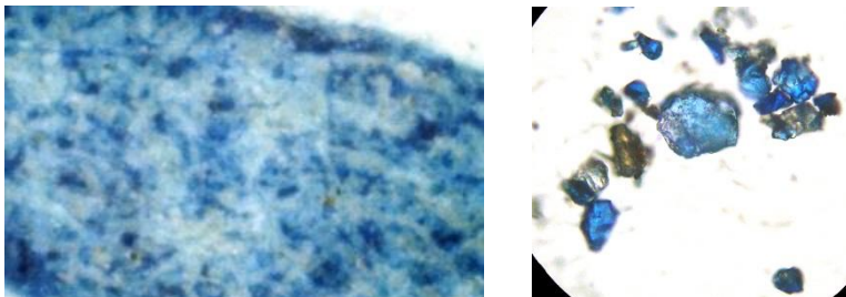
تصویر ۱۴: تصاویر PLM از دو رنگ آبی به کار رفته در نمونه ۲۰ (راست) که لاجورد و نمونه ۱۵ (چپ) که نیل است. بزرگنمایی X400
