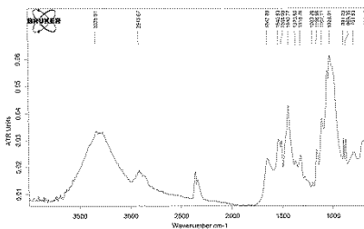
تصویر ۱۹: طیف ATR-FTIR رنگ سفید نمونه ۲۵ که در آن هانتیت شناسایی شد.
