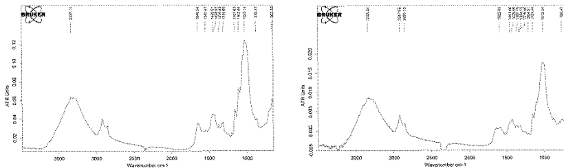
تصویر ۱۰: (راست) طیف ATR- FTIR برگ ۱۷۶، (چپ) طیف ATR- FTIR برگ ۱۰۶
