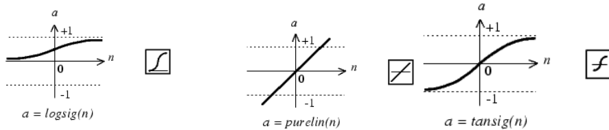
شکل ۴- توابع محرک رایج در شبکه‌های عصبی
