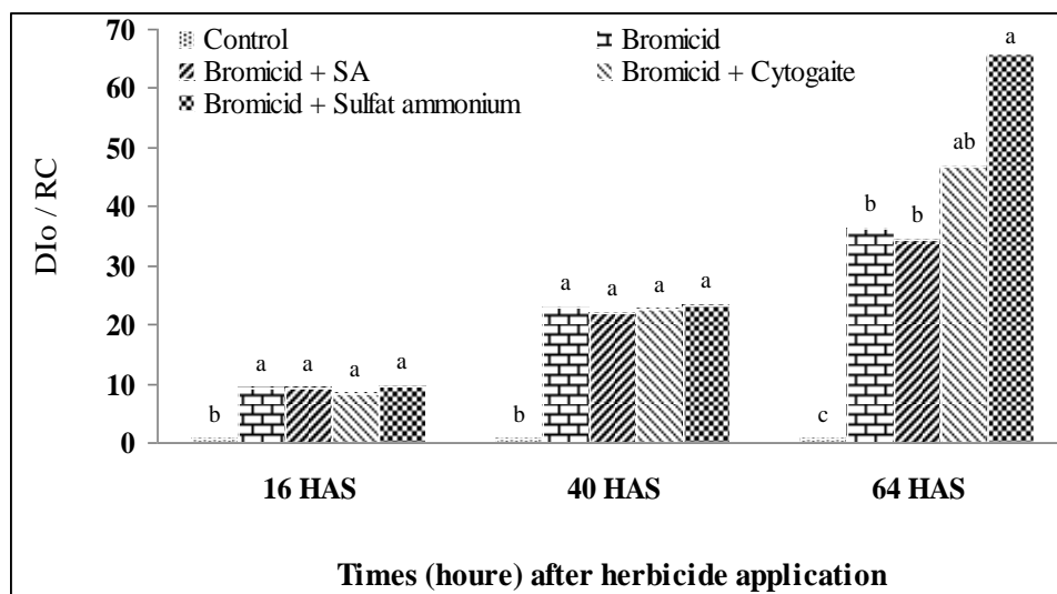
شکل ۵- تأثیر تیمارهای مختلف علف‌کشی بر هدررفت انرژی در هر مرکز واکنش ( DI_0/RC ) تاج خروس ریشه‌قرمز ( Amaranthus retroflexus L.)، ۱۶، ۴۰ و ۶۴ ساعت پس از تیمار. ستون‌های با حروف متفاوت دارای اختلاف آماری معنی‌دار هستند (LSD=5%)
