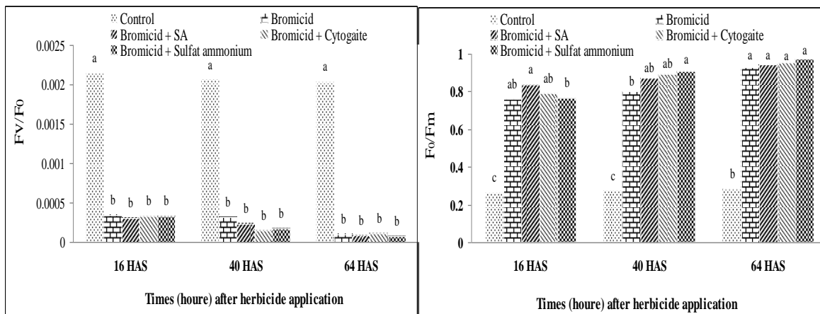
شکل ۳- تأثیر تیمارهای علف‌کشی بر تغییر در پراکندگی گرما در گیرنده‌های فتوسیستم II (F 0 /F m ) و فعالیت کمپلکس تجزیه کننده آب در فتوسیستم II (F v /F 0 ) تاج‌خروس ریشه‌قرمز ( Amaranthus retroflexus L.)، ۱۶، ۴۰ و ۶۴ ساعت پس تیمار. ستون-های با حروف متفاوت دارای اختلاف آماری معنی دار هستند (LSD= 5%)
