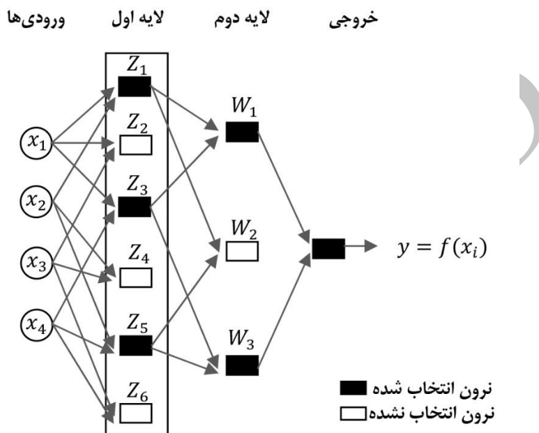
شکل ۱. نمایی از یک شبکه GMDH
