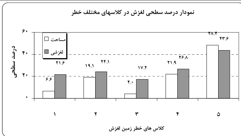
شکل ۷- نمودار توزیع کلاسهای خطر مدل CF برای حوضه شاهد
