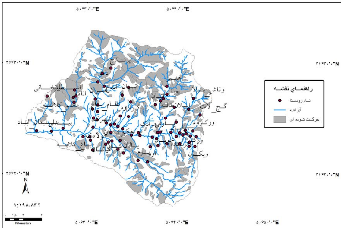
شکل ۲- نقشه پراکنش زمین لغزش‌های حوزه اصلی
