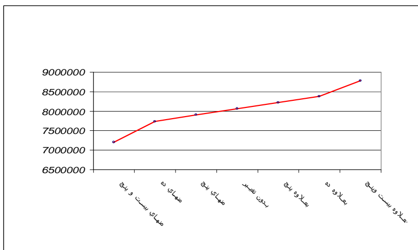
شکل ۷: نمودار خطی روند افزایشی مساحت پهنه سیل گیر با دوره بازگشت ۲۵ ساله و ۱۰، ۵ و ۲۵ درصد افزایش و کاهش ضریب زبری
