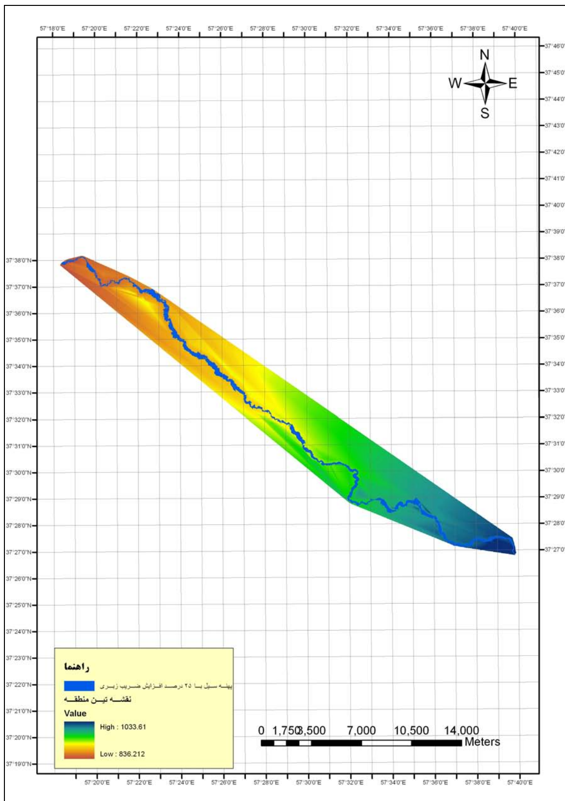
شکل ۴: پهنه بندی سیل با دوره بازگشت ۲۵ ساله و ۲۵ درصد افزایش ضریب زبری
