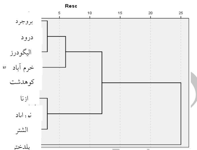
شکل ۲: دندوگرام (نمودار درختی) به روش وارد
