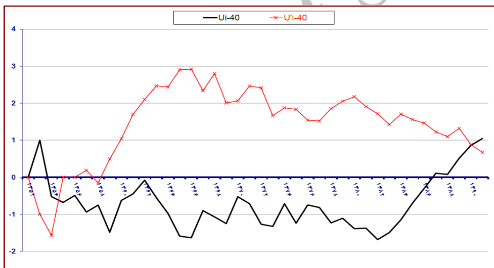
شکل ۱۱: نمودار آزمون معنی‌داری من-کندال سری دامنه‌ی تغییرات مطلق سالانه‌ی دمای روزانه در بازه‌ی ۱۳۹۱-۱۳۵۲ (مأخذ: یافته‌های پژوهش)
