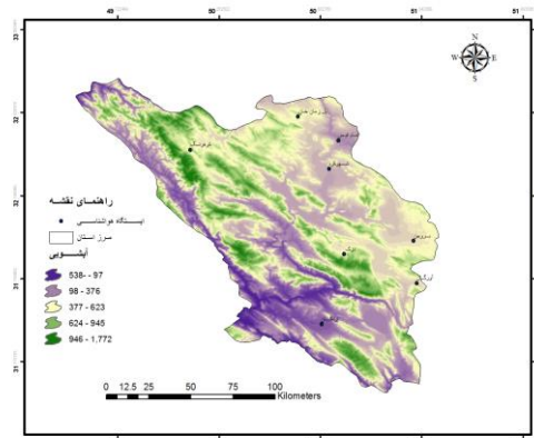
شکل ۸: پهنه‌بندی شاخص‌های رطوبتی
