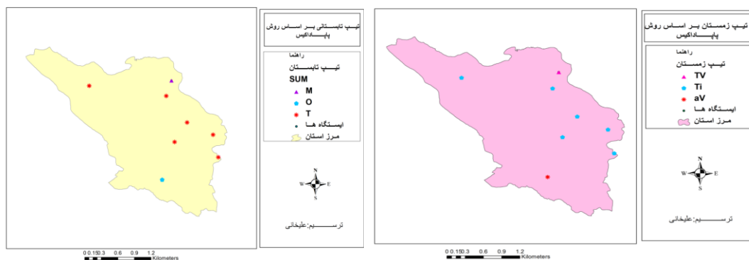
شکل ۳: تیپ زمستانی به روش پاپاداکیس
