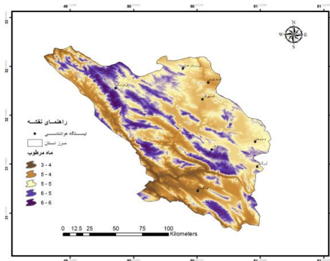
شکل ۶: تعداد ماههای مرطوب
