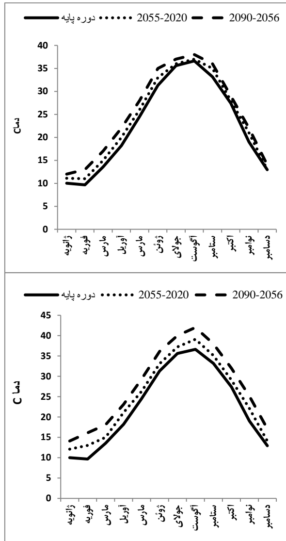
شکل ۴: تغییرات دمای بیشینه ایستگاه ایلام در دوره آینده بر اساس سناریو RCP8.5 و RCP4.5
