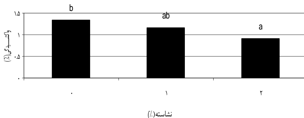
شکل ۸- اثر نشاسته بر واکشیدگی طولی پس از ۲۴ ساعت غوطه‌وری در آب
