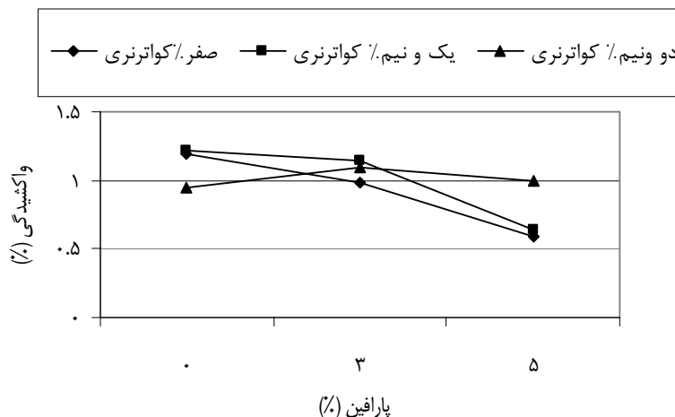
شکل ۷- اثر متقابل پارافین و کواترنری بر واکشیدگی طولی پس از ۲ ساعت غوطه‌وری در آب
