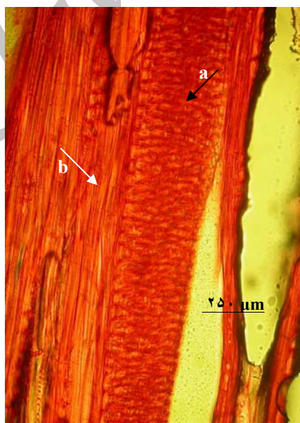
شکل ۸- a. سلول‌های پاراننشیمی اشعه دارای مواد استخراجی قهوه پس از تیمار آب گرمایی b. ترک‌های شعاعی در نزدیکی اشعه‌های پهن و بزرگ
