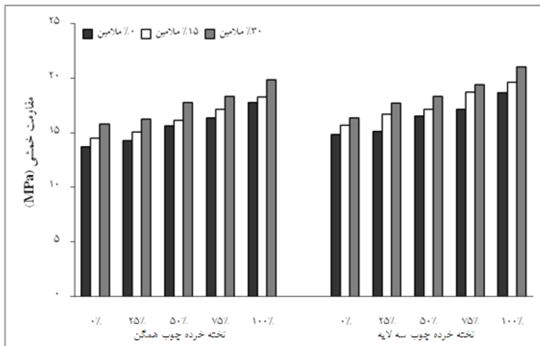
شکل ۱- اثر متقابل درصد اختلاط ساقه کلزا و خرد چوب صنعتی، درصد اختلاط چسب ملامین با اوره فرمالدهید و نوع تخته بر مقاومت خمشی تخته‌خرد چوب
