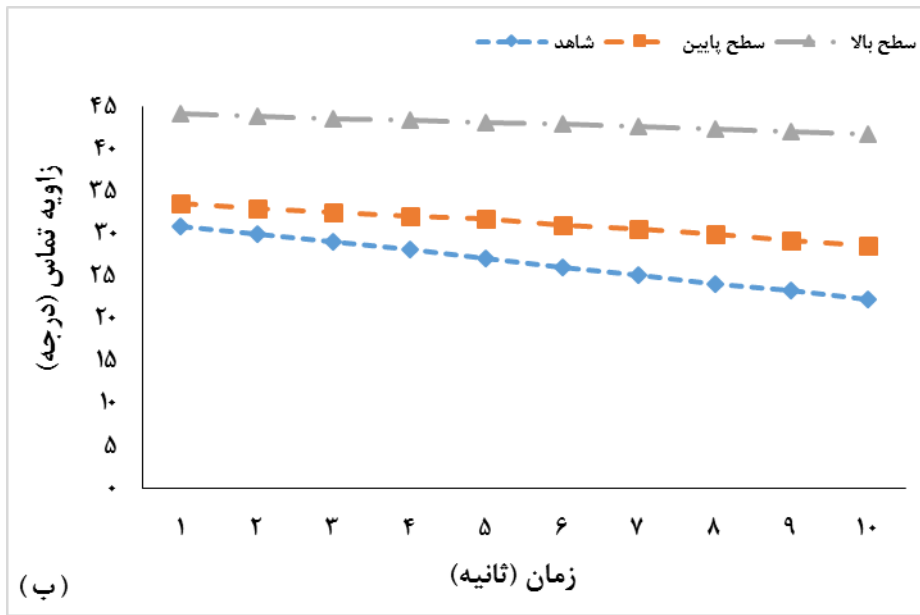
شکل ۳- تأثیر میزان فورفوریلایسیون بر زاویه تماس قطره در آزمون‌های چوب راش (الف) و نراد (ب)
