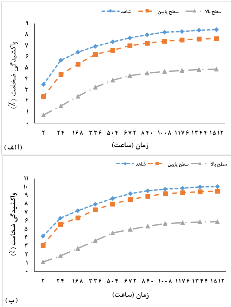
شکل ۲- تأثیر میزان فورفوریل‌اسیون بر درصد واکسیدگی ضخامت چوب راش (الف) و نراد (ب)
