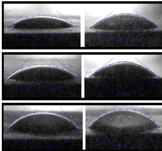
شکل ۴- زاویه تماس قطره در سطوح مختلف فورفوریلایسیون در ثانیه اول (سمت راست گونه راش و چپ گونه نراد، ردیف اول تا سوم به ترتیب آزمون‌های شاهد، سطح پایین و سطح نسبتاً بالای فورفوریلایسیون)
