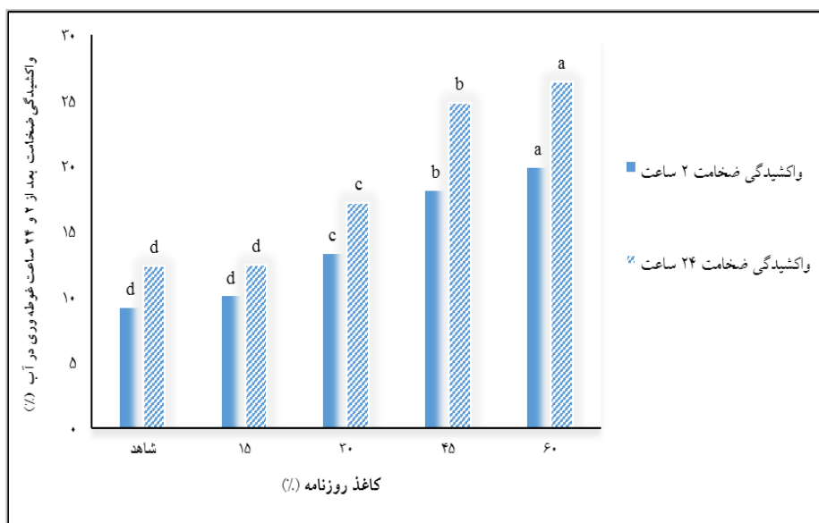
شکل ۷- اثر سطوح مختلف کاغذ روزنامه باز یافتی بر واکنشیدگی ضخامت بعد از ۲ و ۲۴ ساعت غوطه‌وری در آب
