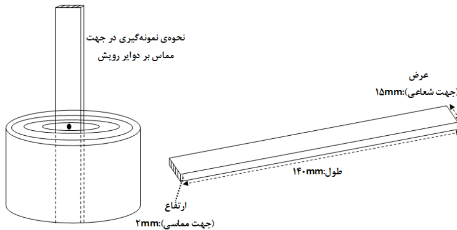
شکل ۲- نحوه‌ی تهیه نمونه‌های آزمونی جهت آزمون ارتعاش اجباری خمشی
