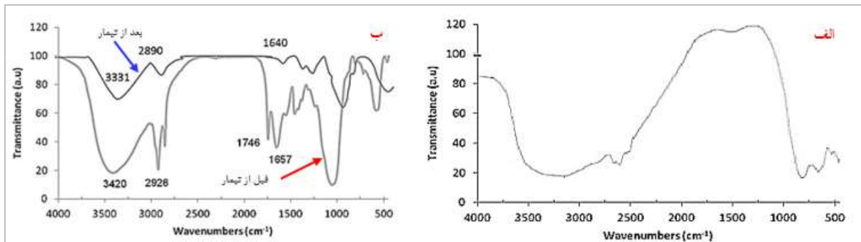
شکل ۵- طیف FTIR الف) جلبک ضایعاتی اسپیرولینا، ب) الیاف سلولزی قبل و بعد از خالص سازی تصاویر SEM
