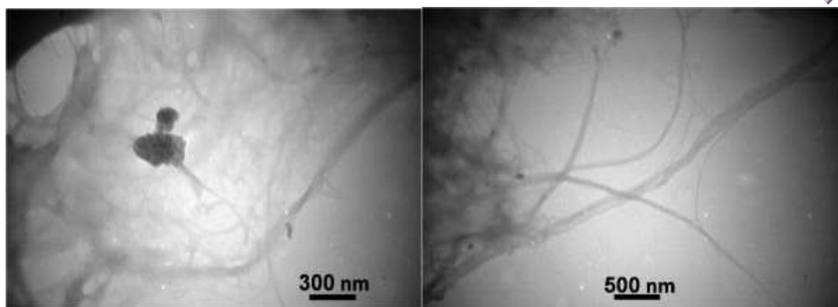
شکل ۱- تصویر TEM از نانوالیاف لیگنوسلولوز حاصل از کارتن‌های کنگره‌ای کهنه
