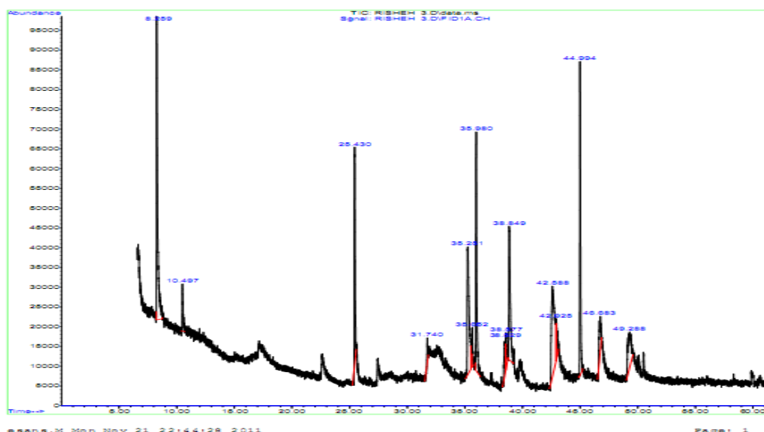
شکل ۸- کروماتوگرام گازی ترکیبات شیمیایی عصاره چوب ریشه درختچه دیودال با حلال استن
