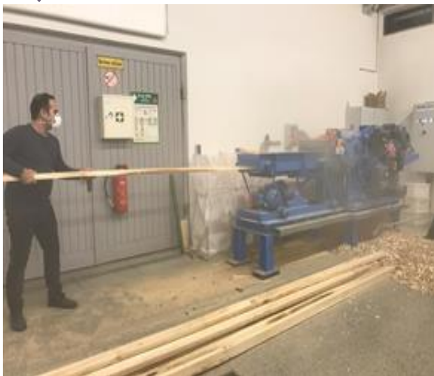
شکل ۲- خردکن استوانه‌ای در حین تولید چپیس
