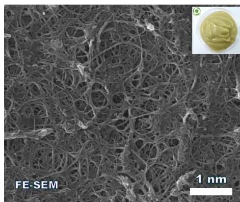
شکل ۳- تصویر FE-SEM ژل نانوکیتوزان تولید شرکت نانونین پلیمر
