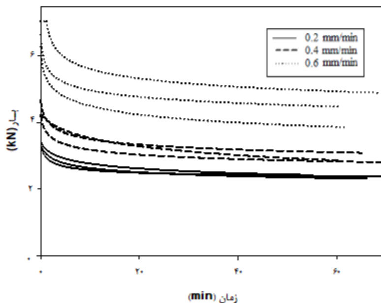
شکل ۱- منحنی‌های افت تنش چوب فشرده در سه سطح سرعت بارگذاری
