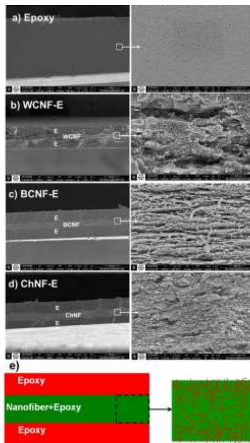
شکل ۲- ریزنگاره FE-SEM از سطح مقطع شکست کششی نمونه‌ها به همراه مدل شماتیک سطح مقطع نانوکامپوزیت سه‌لایه
