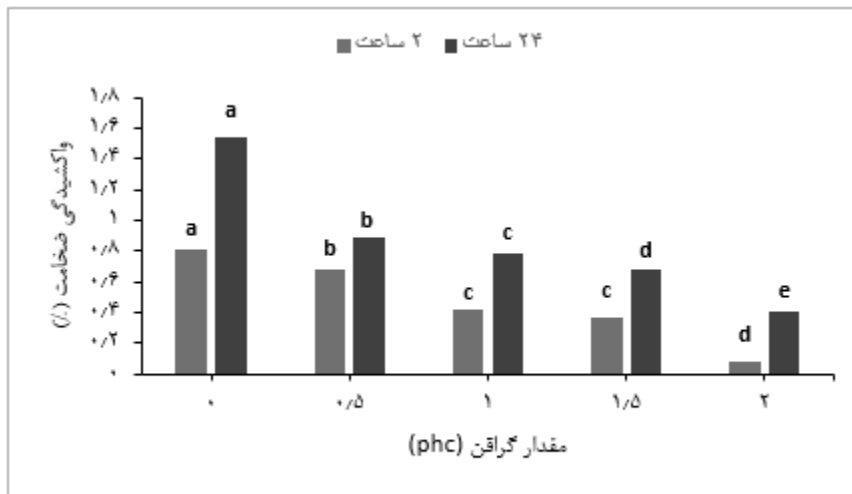
شکل ۱۲- تاثیر نانوغرافن بر میزان واکنشیدگی ضخامت چندسازه حاصل از آرد ساقه کلزا- پلی اتیلن سنگین
