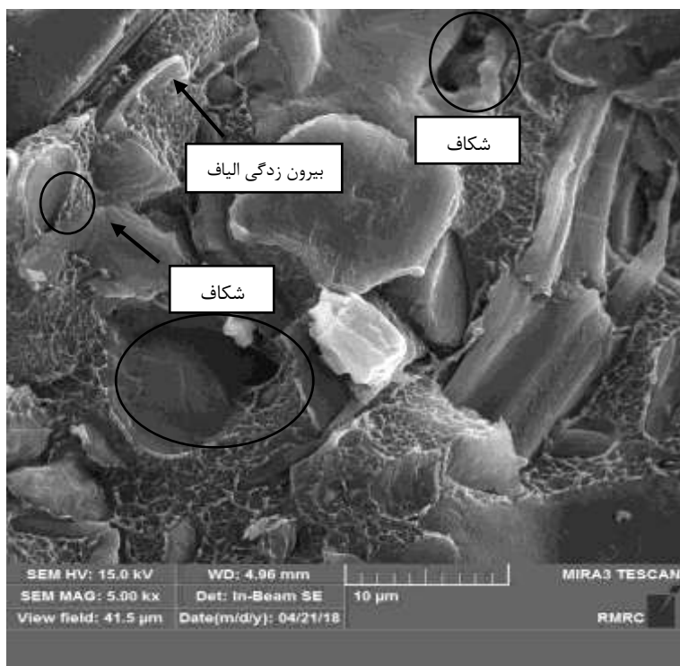
شکل ۱- تصویر میکروسکوپ الکترونی FESEM نانو چندسازه حاصل از آرد ساقه کلزا- پلی اتیلن سنگین (فاقد نانوگرافن)
