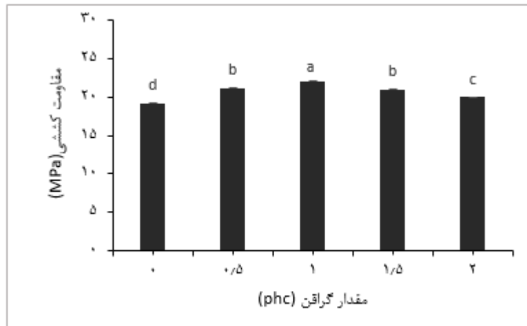
شکل ۸- تاثیر نانوگرافن بر میزان مقاومت کششی چندسازه حاصل از آرد ساقه کلزا- پلی اتیلن سنگین
