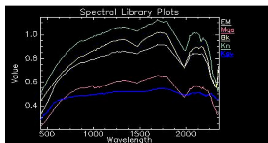
شکل ۶. طیف استخراج‌شده از تصویر مربوط به واحدهای سنگی منطقه مورد مطالعه
