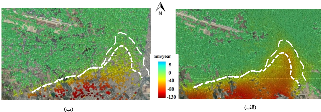
شکل ۷. نقشه تغییرات. الف) نقشه نرخ تغییرات منطقه مطالعاتی حاصل از تحلیل تداخل سنجی مجموعه داده مسیر ۳۵ S-1A؛ ب) نقشه نرخ تغییرات منطقه مطالعاتی حاصل از تحلیل تداخل سنجی مجموعه داده مسیر ۱۴۹ ENVISAT-ASAR
