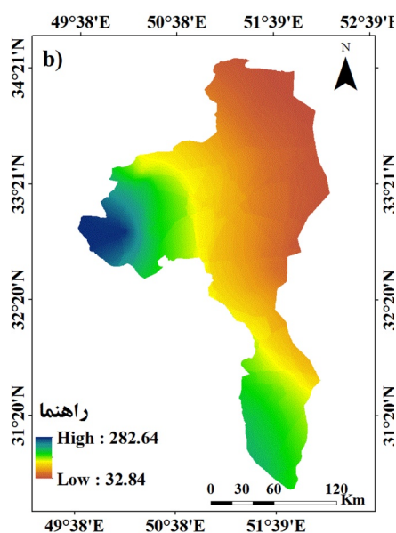
شکل ۶. میزان شاخص RUE (g C/m2 y-1/mm) و بارش (a) و سالیانه (b) در مناطق نیمه‌استپی استان اصفهان
