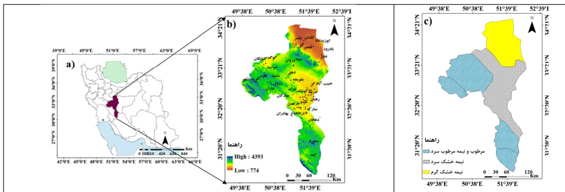
شکل ۱. موقعیت جغرافیایی منطقه مورد مطالعه (a)، نقشه رقوم‌اری (b)، نقشه طبقات اقلیمی (c)
