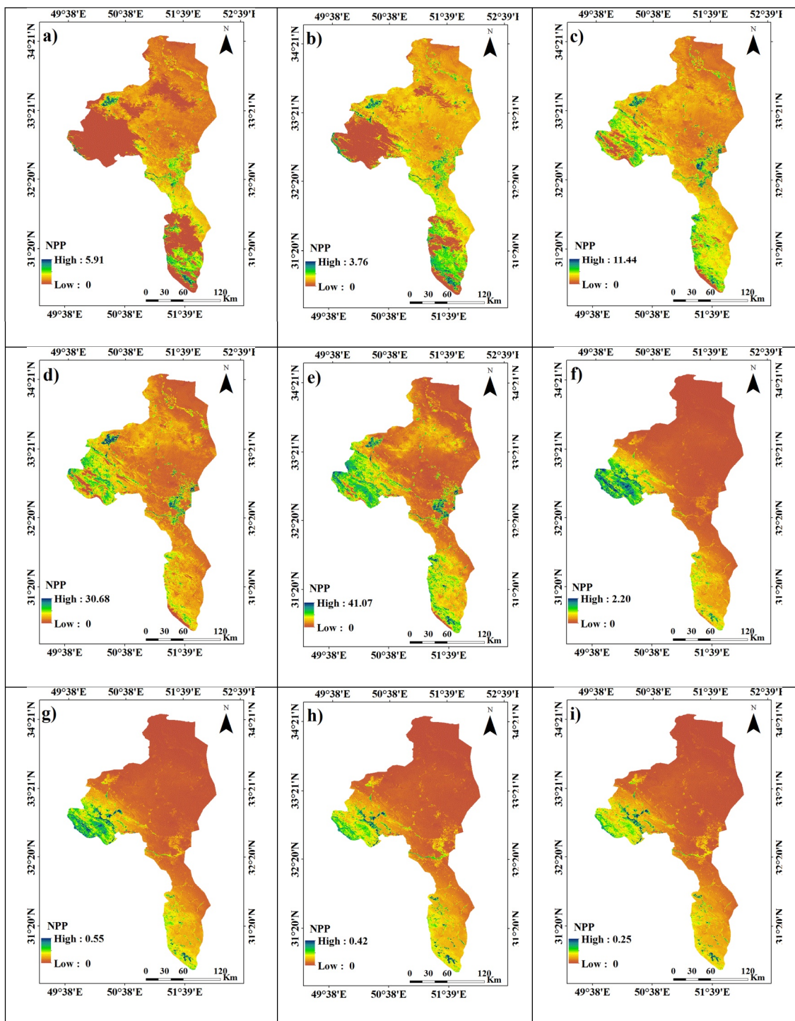
شکل ۳. مقادیر ماهیانه تولید خالص اولیه بر حسب C/m^2/mo ، در سال ۲۰۱۶ ، ژانویه (دی) (a)، فوریه (بهمن) (b)، مارس (سفند) (c)، آوریل (فروردین) (d)، می (اردیبهشت) (e)، ژوئن (خرداد) (f)، ژوئیه (تیر) (g)، آگوست (مرداد) (h)، سپتامبر (شهریور) (i)، اکتبر (مهر) (j)، نوامبر (آبان) (k)، دسامبر (آذر) (l) و مقدار NPP سالیانه ( C/m^2 y^{-1} ) (m)
