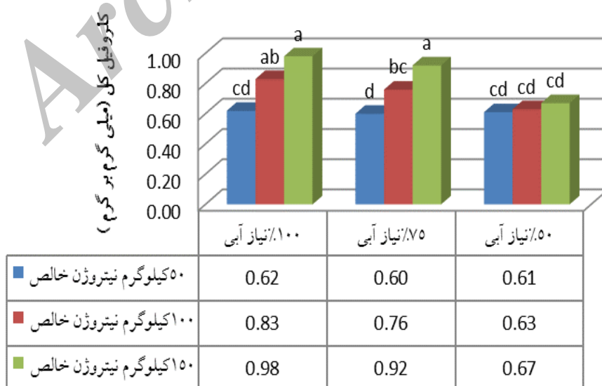
شکل ۱- مقایسه میانگین اثر متقابل کم آبیاری و نیتروژن بر میزان کلروفیل کل برگ
