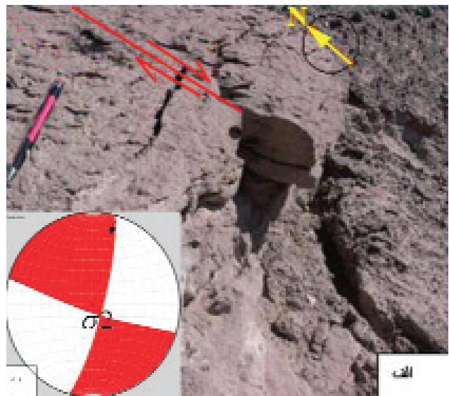
تصویر ۲-الف- قسمتی از گسل راست بر کهورک، ب- استریوگرام مربوط به آن که راست بر بودن آن را نشان می‌دهد.
