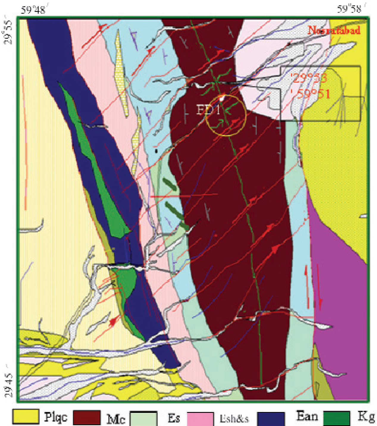
تصویر ۱- نقشه‌ی زمین‌شناسی ساده شده از منطقه‌ی نصرت آباد. گسل نصرت آباد دارای سازوکار امتدادلغز با مؤلفه‌ی معکوس می‌باشد. واحد: Mc کنگلومرای کنجی که دچار چین خوردگی شده است.
