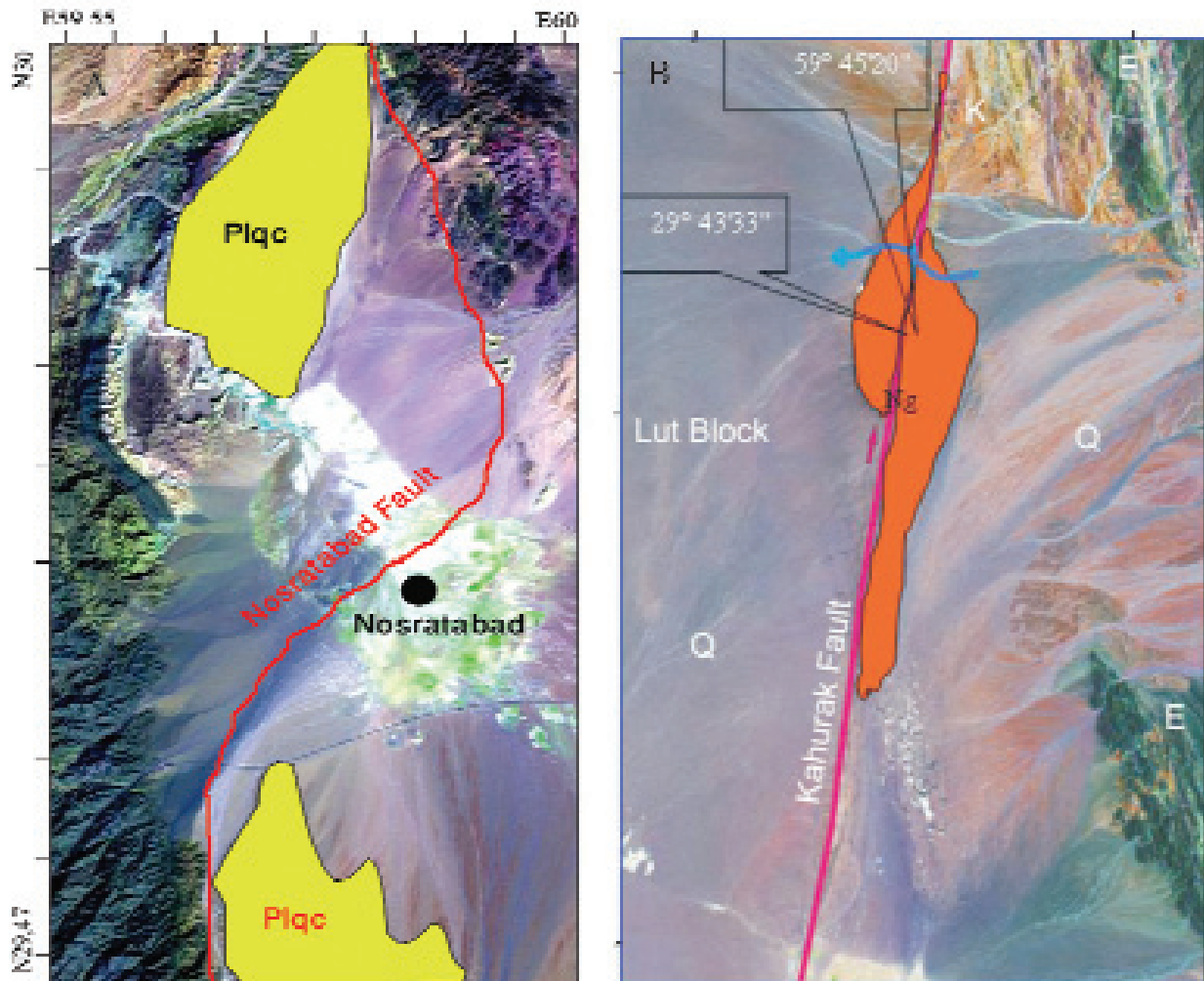
تصویر ۳-۱-۳-۲-۱-۴-۷ از گسل نصرت آباد که نشان می‌دهد این گسل نهشته‌های پلیو-کواترنری را حدود ۱۰ کیلومتر جابه‌جا نموده است. B- گسل کهورک، بیانگر جابه‌جایی راست بر نهشته‌های نئوژن به اندازه‌ی ۷ کیلومتر و یک آبراهه به اندازه‌ی ۱ کیلومتر است.
