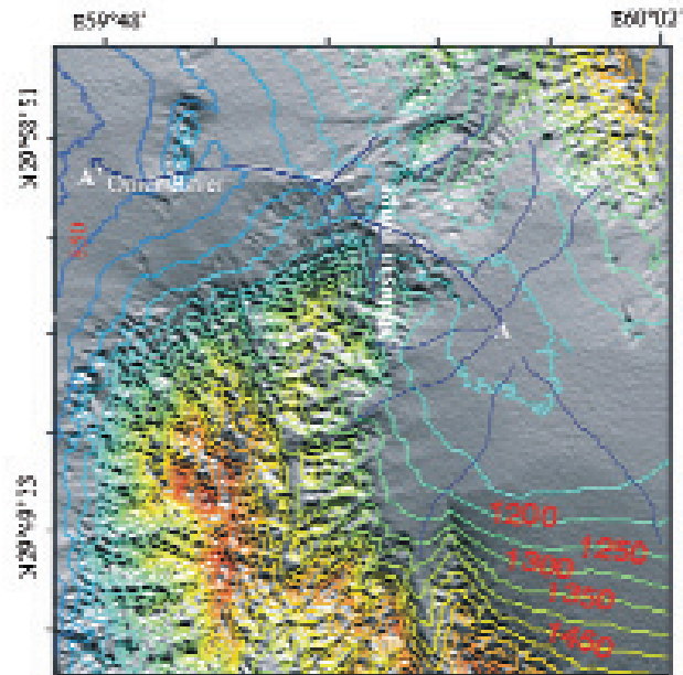
تصویر ۶- تصویر اس آر تی ام (SRTM) از منطقه‌ی نصرت آباد که به وسیله‌ی نرم‌افزاری آر-مپر نقشه‌ی توپوگرافی ۱/۱۰۰۰۰ تهیه گردیده است. این تصاویر دارای بعد ارتفاعی می‌باشند که در تهیه‌ی نقشه‌های توپوگرافی مورد استفاده قرار می‌گیرند. در این تصویر حوضه‌های آبریز رود عمر مشاهده می‌گردند. A و A' مسیر مقطع عرضی تصویر ۷ را نشان می‌دهند.
