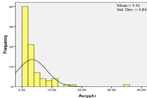
تصویر ۹- هیستوگرام فراوانی عنصر طلا
