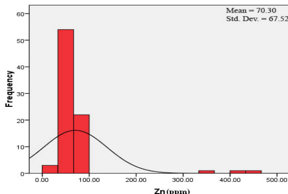
تصویر ۱۳- هیستوگرام فراوانی عنصر روی
