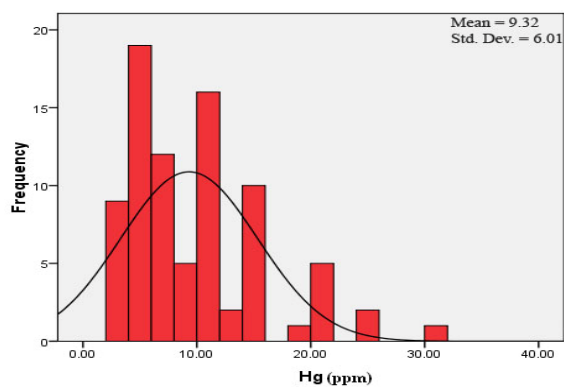
تصویر ۱۶- هیستوگرام فراوانی عنصر جیوه
