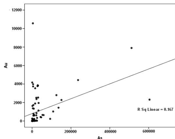
تصویر ۱۷- نمایش پراکنش عنصر طلا با عنصر آرسنیک به همراه منحنی رگرسیون
