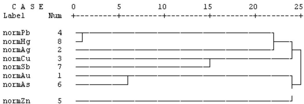
تصویر ۱۹- دندروگرام مربوط به رسوبات آبراهه‌ای
