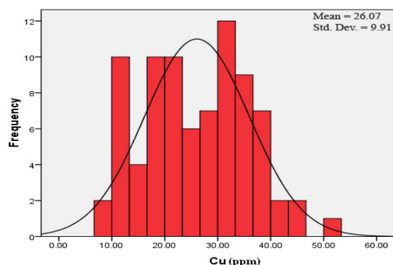
تصویر ۱۱- هیستوگرام فراوانی عنصر مس
