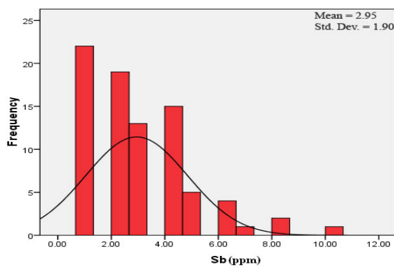
تصویر ۱۵- هیستوگرام فراوانی عنصر آنتیموان
