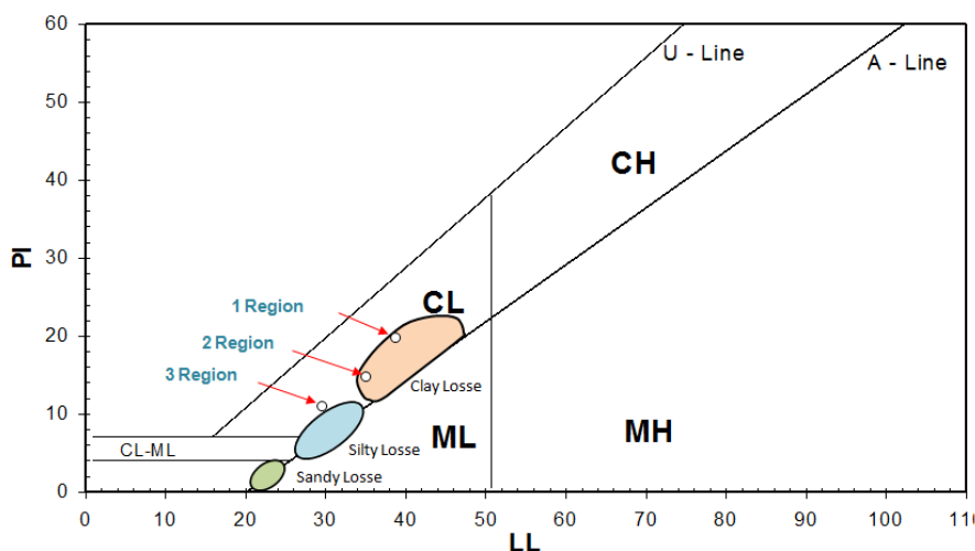
تصویر ۹- موقعیت لس‌های استان در نمودار خمیری
