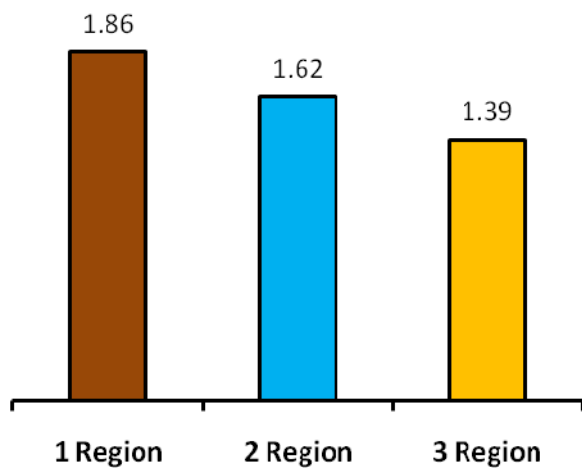
تصویر ۶- مقادیر دانسیته خشک طبیعی برای لس‌های استان در سه ناحیه
