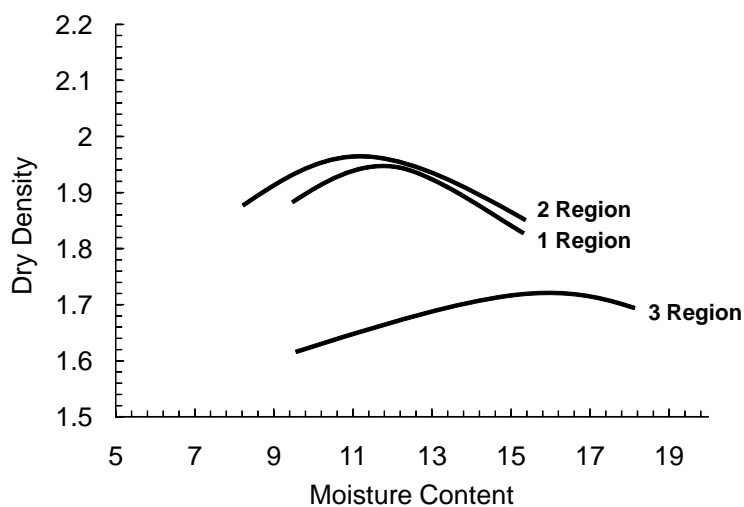
تصویر ۱۴- تغییرات منحنی تراکم در لس‌های سه ناحیه
