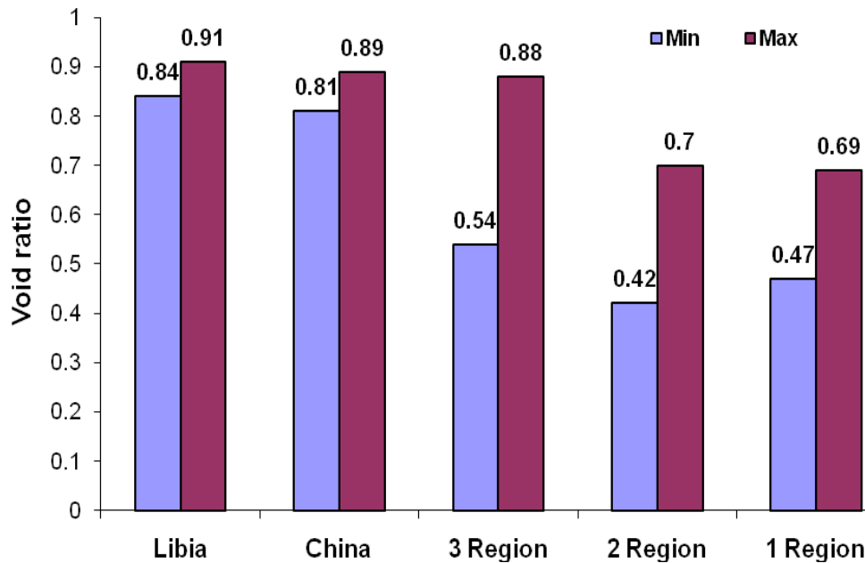
تصویر ۱۰- مقایسه نسبت پوکی لس‌های استان با لس‌های چین و لیبی
