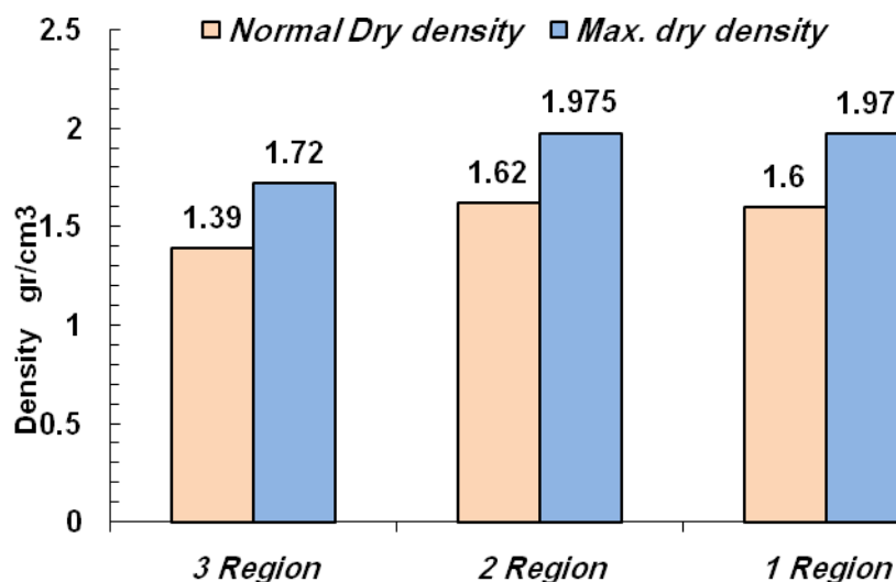
تصویر ۱۱- مقایسه دانسیته خشک طبیعی و دانسیته حداکثر لس‌های سه ناحیه استان
