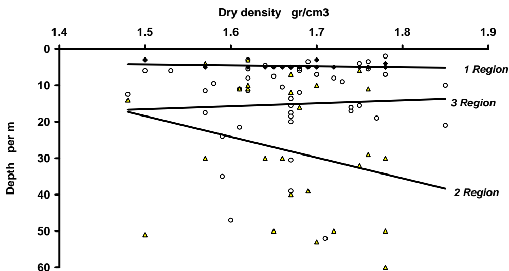
تصویر ۷- تغییرات دانسیته نسبت به عمق در لس‌های استان
