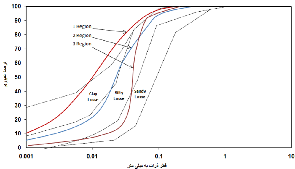
تصویر ۵- متوسط دانه‌بندی لس‌های سه ناحیه در پوش دانه‌بندی
