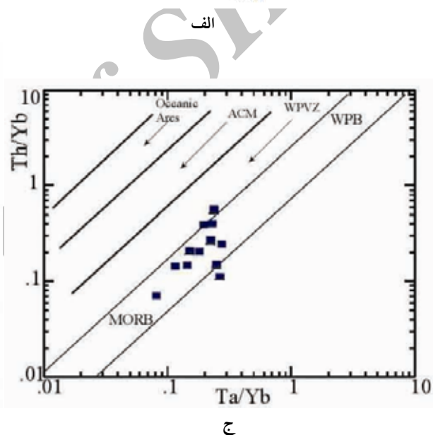
تصویر ۶- الف- نمودار تقسیم بندی سنگها بر مبنای Zr/TiO_2 در برابر Nb/Y (وینچستر و فلویید ۱۹۷۷) ب- نمودار مثلثی FeO-Na_2O+K_2O-MgO (ایرون و باراگار ۱۹۷۱) ج- نمودار Th/Yb در مقابل Ta/Yb (پیرس ۱۹۸۳). د- نمودار Zr/Y - Zr متمایز کننده بازالتها (فلویید و همکاران ۱۹۹۱)
