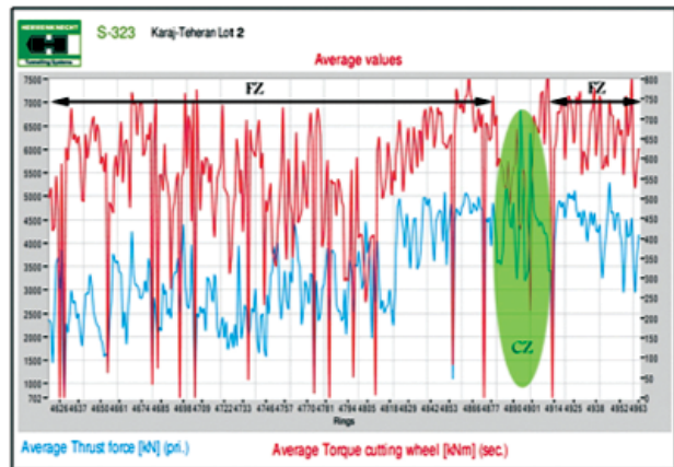
تصویر ۱۱- تغییرات متوسط گشتاور و نیروی پیشران در زون گسله پورکان-
