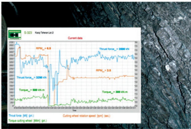
تصویر ۱۰- توده سنگ نازک لایه و سست سینه کار در متر ۶۳۶۵ و پارامترهای ثبت شده برای آن
