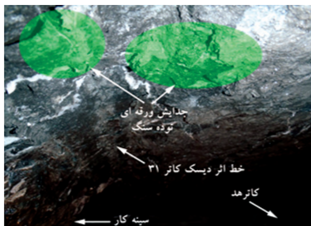
تصویر ۷- سقف تونل در جلوی کاترهد و در محل گسل پورکان
