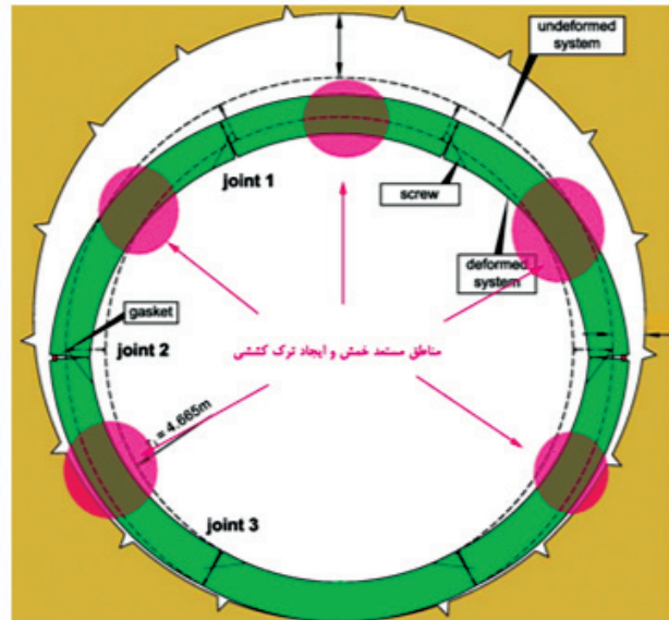
تصویر ۵- محدوده های مستعد ایجاد ترک کششی در یک رینگ تخم مرغی
