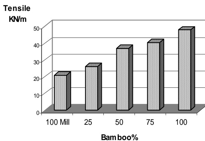
شکل 4- مقایسه مقاومت کششی کاغذ حاصل از خمیر CMP بامبو و خمیر CMP کارخانه
