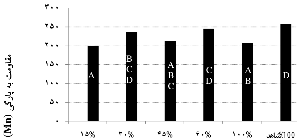
نسبت ترکیب خمیر بید شکل ۴- میزان مقاومت به پارگی کاغذهای دست ساز
