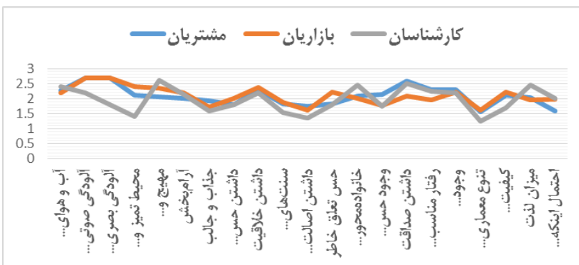
شکل شماره ۱: مقایسه میانگین تأثیرگذاری شاخص‌های متغیر تصویر مقصد بازار از نظر سه گروه آماری
