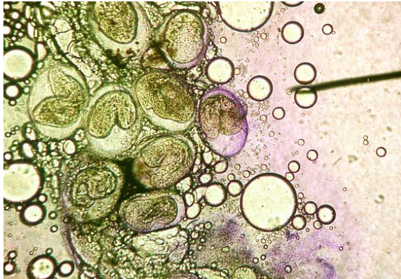
شکل ۲- تجمع کیست انگل Alloceradium sp. در کیسه هوایی ماهی برگ‌بیدی رودخانه فهلیان (درشت‌نمایی \times 800 ).
