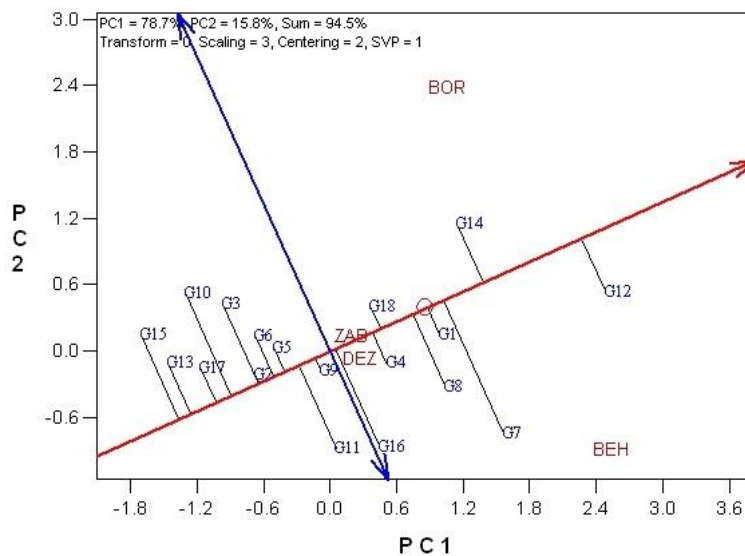
شکل ۶- بردار محیط متوسط (AEC) پایداری عملکرد دانه ژنوتیپهای کلزا به روش تجزیه گرافیکی GGE بای پلات در محیطهای آزمون مختلف
