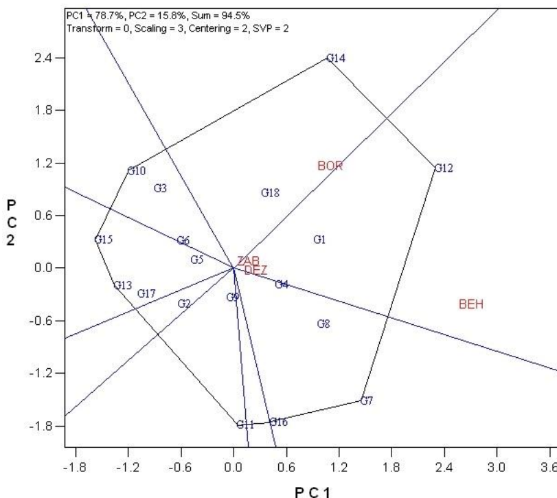
شکل ۱- تجزیه گرافیکی بای‌پلات و نمایش الگوی کدام-برتر-کجا بر اساس میانگین عملکرد دانه ژنوتیپ‌های کلزا در محیط‌های آزمون مختلف
