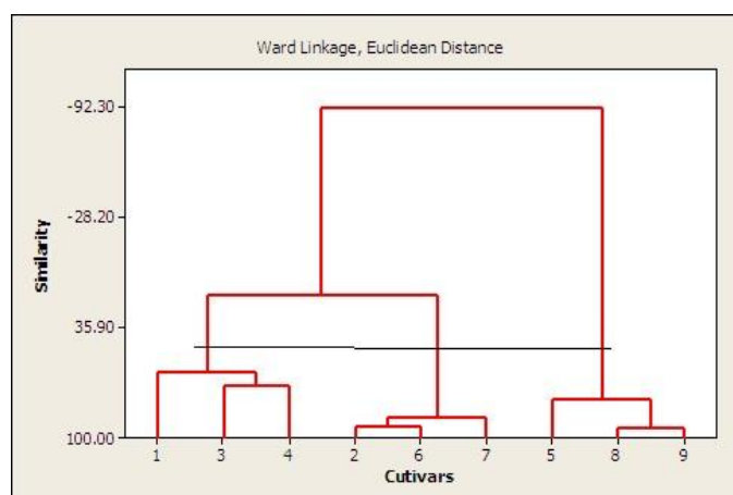
شکل ۲- تجزیه خوشه‌ای ارقام گندم با استفاده از روش ward (۱- مهدوی، ۲- آذر ۲، ۳- کویر، ۴- روشن، ۵- قدس، ۶- اکسکلیبر، ۷- کل حیدری، ۸- شیراز و ۹- شاه‌پسند) Figure 2. The cluster analysis of bread wheat cultivars according to ward method (1. Mahdavi, 2. Azar2, 3. Kavir, 4. Roushan, 5. Ghods, 6. Excaliber, 7. Kalheydari, 8. Shiraz and 9. Shahpasand).
