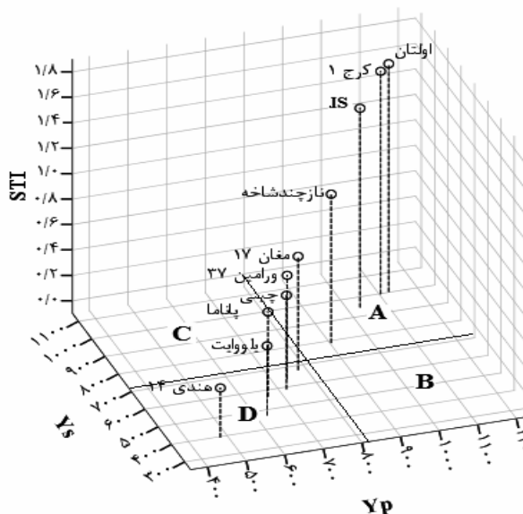
شکل 1- نمودار تعیین ارقام متحمل به خشکی براساس عملکرد در شرایط تنش و بدون تنش و شاخص STI در شرایط آبیاری به مقدار 75 درصد نیاز آبی گیاه (الف) و در شرایط آبیاری به مقدار 50 درصد نیاز آبی گیاه (ب).
