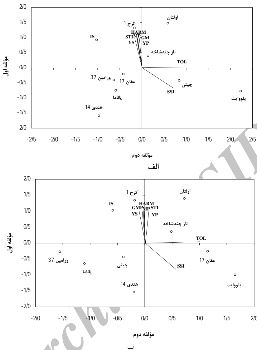
شکل 2- بای پلات 10 رقم کنجد و هشت شاخص تحمل به خشکی بر اساس اولین و دومین مؤلفه اصلی در شرایط آبیاری به مقدار 75 درصد (الف) و 50 درصد (ب) نیاز آبی
