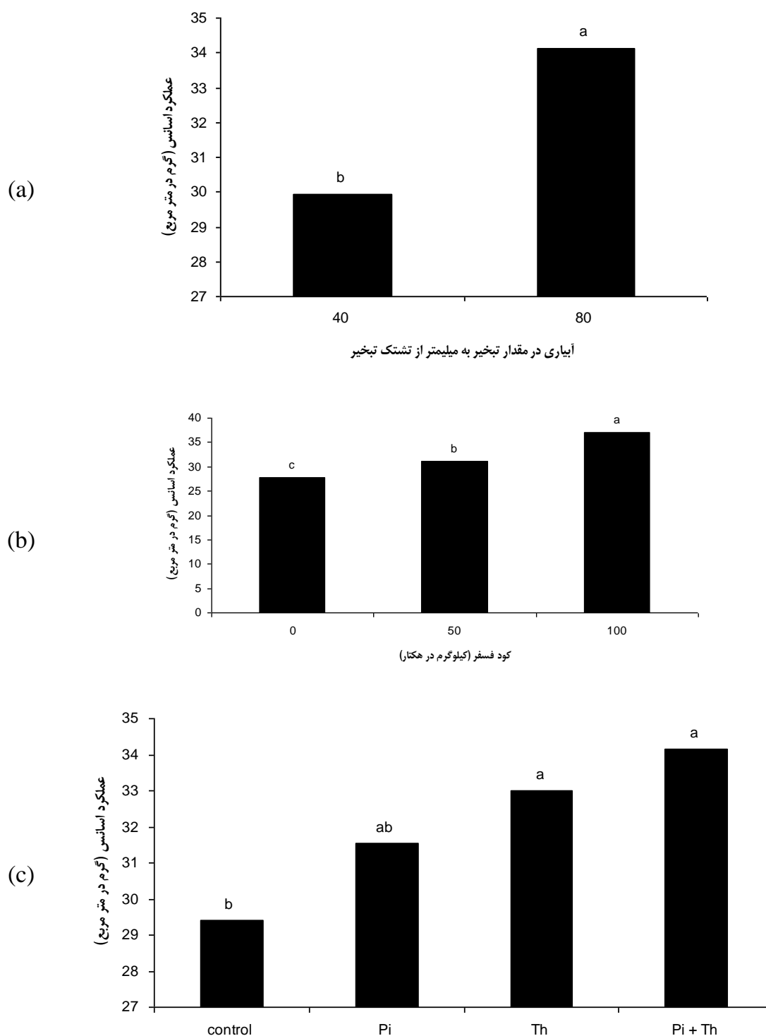
شکل ۴- اثر سطوح آبیاری (a)، کود فسفر (b) و تیمارهای قارچ (c) بر عملکرد اسانس نعناع فلفلی
