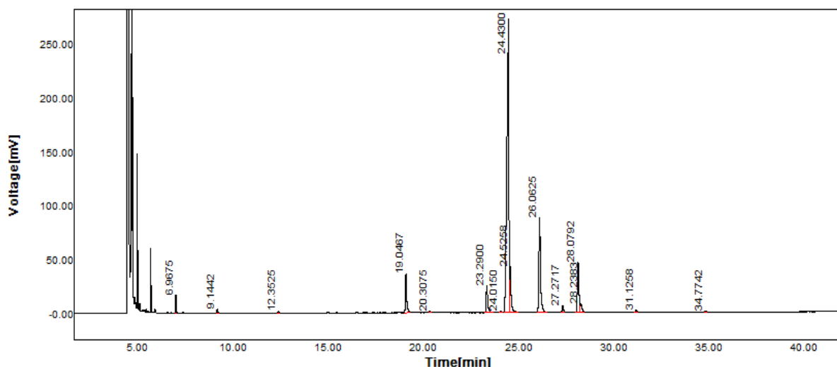
شکل ۱- کروماتوگرافی گازی حاصل از متیل استرهای اسیدهای چرب روغن دانه در تیمار شاهد بدون تلقیح گیاه کلزا
