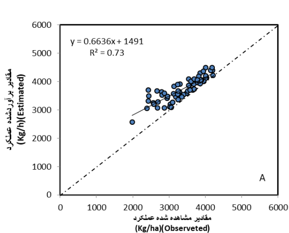
شکل ۲- مقایسه مقادیر عملکرد واقعی و شبیه‌سازی شده با مدل WOFOST در سال ۱۳۹۱. برای ارقام بومی (A) و ارقام پرمحصول (B)
