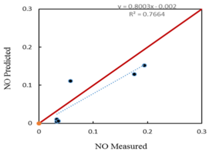
شکل ۳- مقایسه مقادیر اندازه‌گیری و برآورد شده اکسید نیتریک بر مبنای مدل DAYCENT
